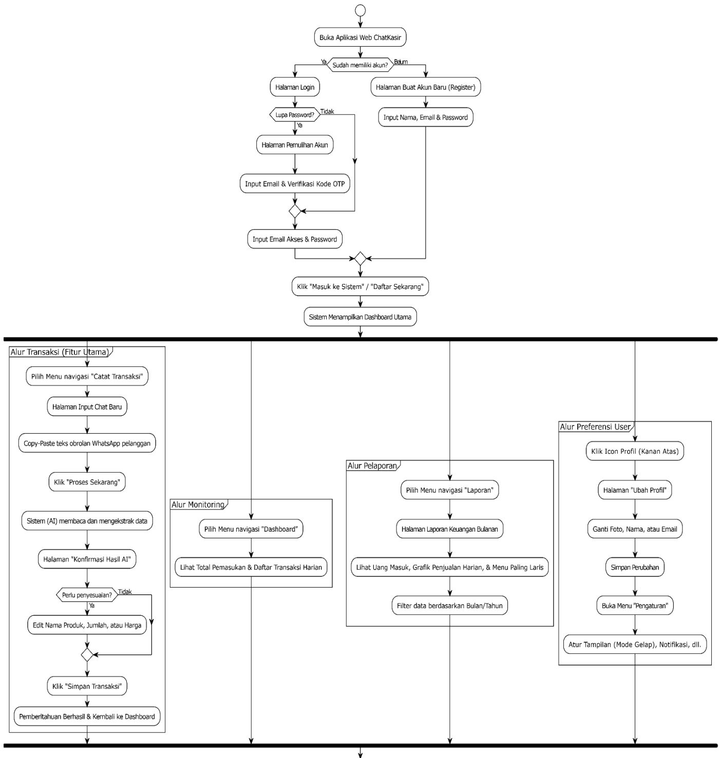
Flowchart Alur Pengguna (User Flow) - ChatKasir
